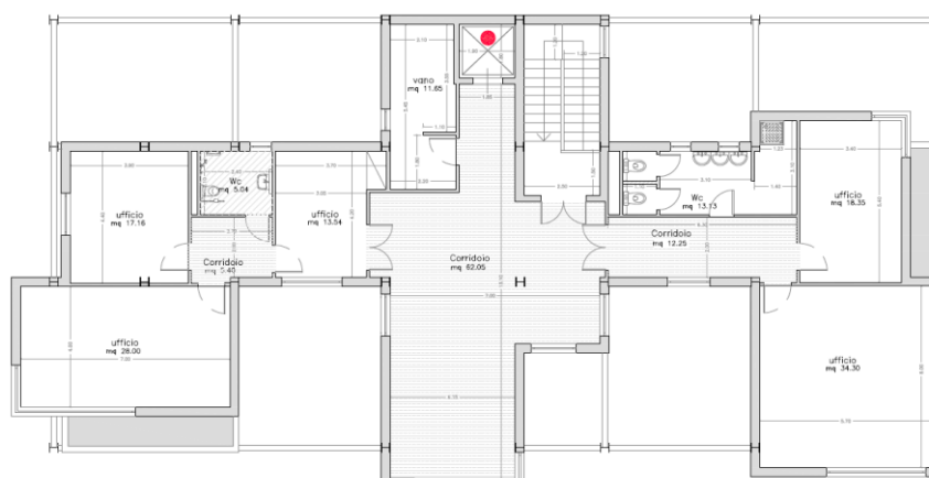
PIANO PRIMO RAPP. 1:100
